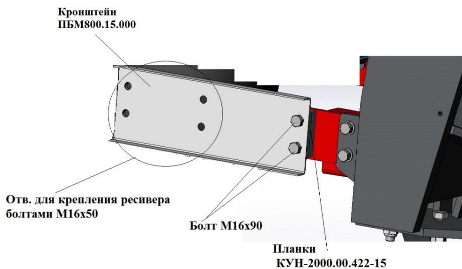
Рис.9 Установка ресивера
