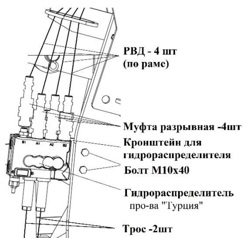
Рис.8 Установка гидрораспределителя
